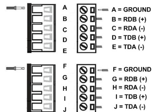
RS-422 / Four Wire RS-485
